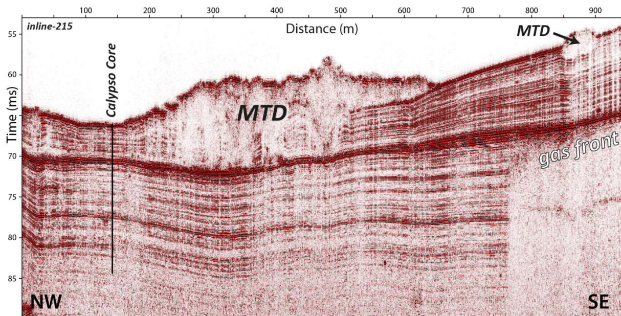
Figur 17. Seismisk profil fra Finneidfjord. Gas er indikert under markerte refleksjoner som representerer et spesielt leirlag i fjordbunnen (dokumentert av kjerne (calypso core: GS10-163-02), se også Figur 25). Skredavsetninger er indikert (MTD: mass transport deposit). Omarbeidet fra Vanneste m.fl. (2012).
