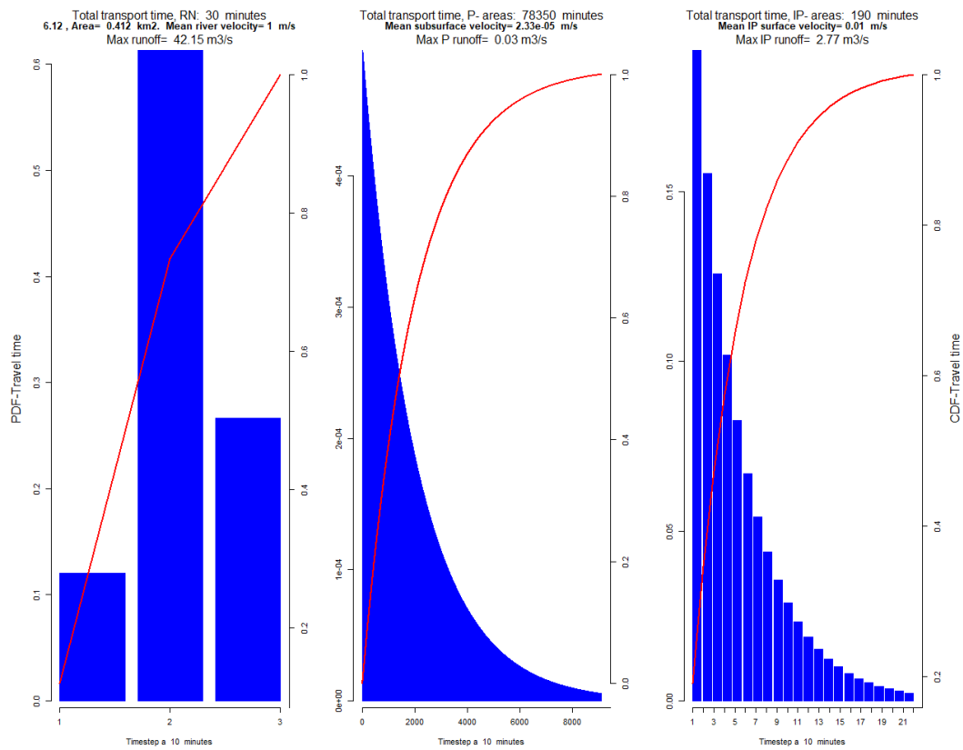
Figur 4 Reisetidsfordelinger for 6.12 Vestli, 10 minutters tidsopløsning. Reisetidsfordeling i elvenettverket (til venstre), til P-arealer (i midten) og for IP-arealer (til høyre). Blå søyler viser histogram av reisetidsfordeling (fraksjon per tidskritt), og rød linje viser kumulativ reisetidsfordeling.
